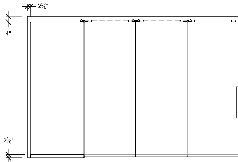
Double glazed left stacking system with integrated handle Système à verre double empiage à gauche avec poignée intégrée
