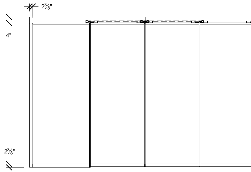
Single glazed left stacking system with integrated handle Système à verre simple empilage à gauche avec poignée intégrée
