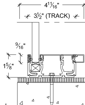
Trim on office side of a single 1/2" glass wall Ornement côté bureau d'un mur simple en verre de 1/2 po
