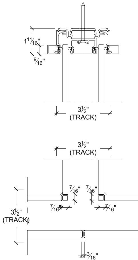
Double glazed T condition Retour en T verre double
