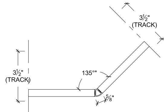
1/2" polycarbonate for variable angle condition Polycarbonate pour condition en angle variable 1/2 po
