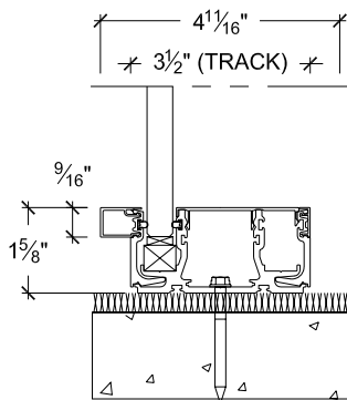
Trim on corridor side of a single 1/2" glass wall Ornement côté couloir d'un mur simple en verre de 1/2 po
